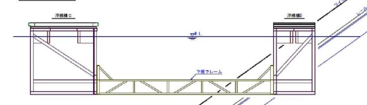
浮桟橋正面図
