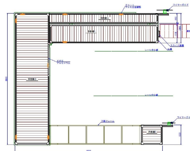
浮桟橋平面図
